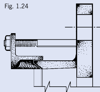
Brida de diámetro especial "S"
