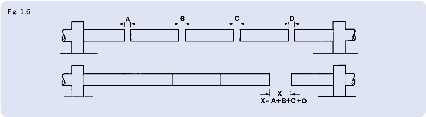
a) Tuberías tendidas en línea recta con holguras de instalación iguales. b) La holgura acumulada (X) en una tubería recta no debe exceder el valor máximo permisible que se indica en la Tabla de holguras de instalación.
