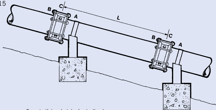
Soporte típico de tuberías inclinadas.
