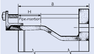
Cuerpo central prolongado
