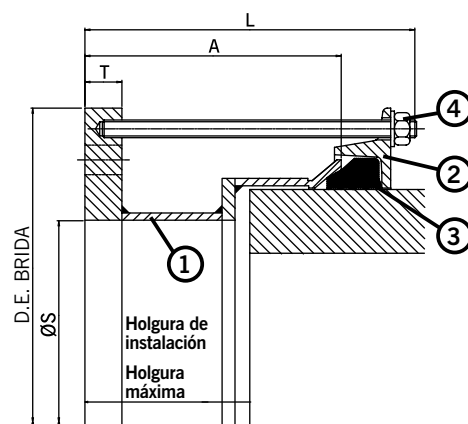
Adaptador de brida de Tipo 3
