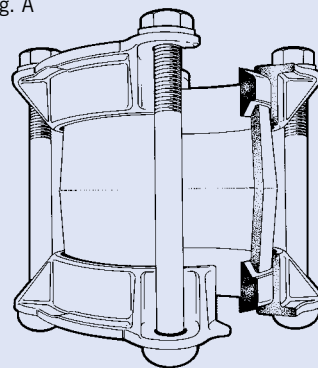
Ilustración de la sección de una unión recta Viking Johnson.
