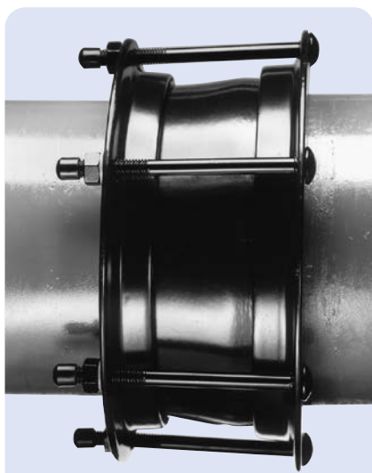
Unión reducida con manguito prolongado
