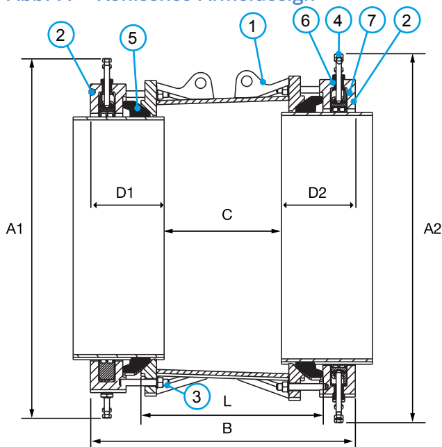
Abb. A – Konisches Ärmel-Design
