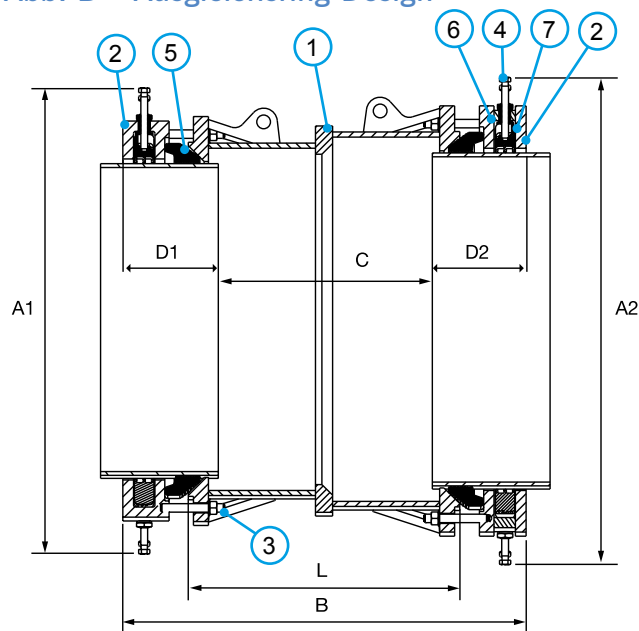
Abb. B – Ausgleichsring-Design
