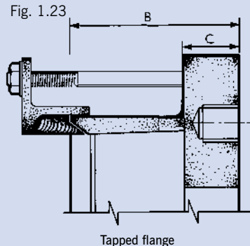
Tapped flange
